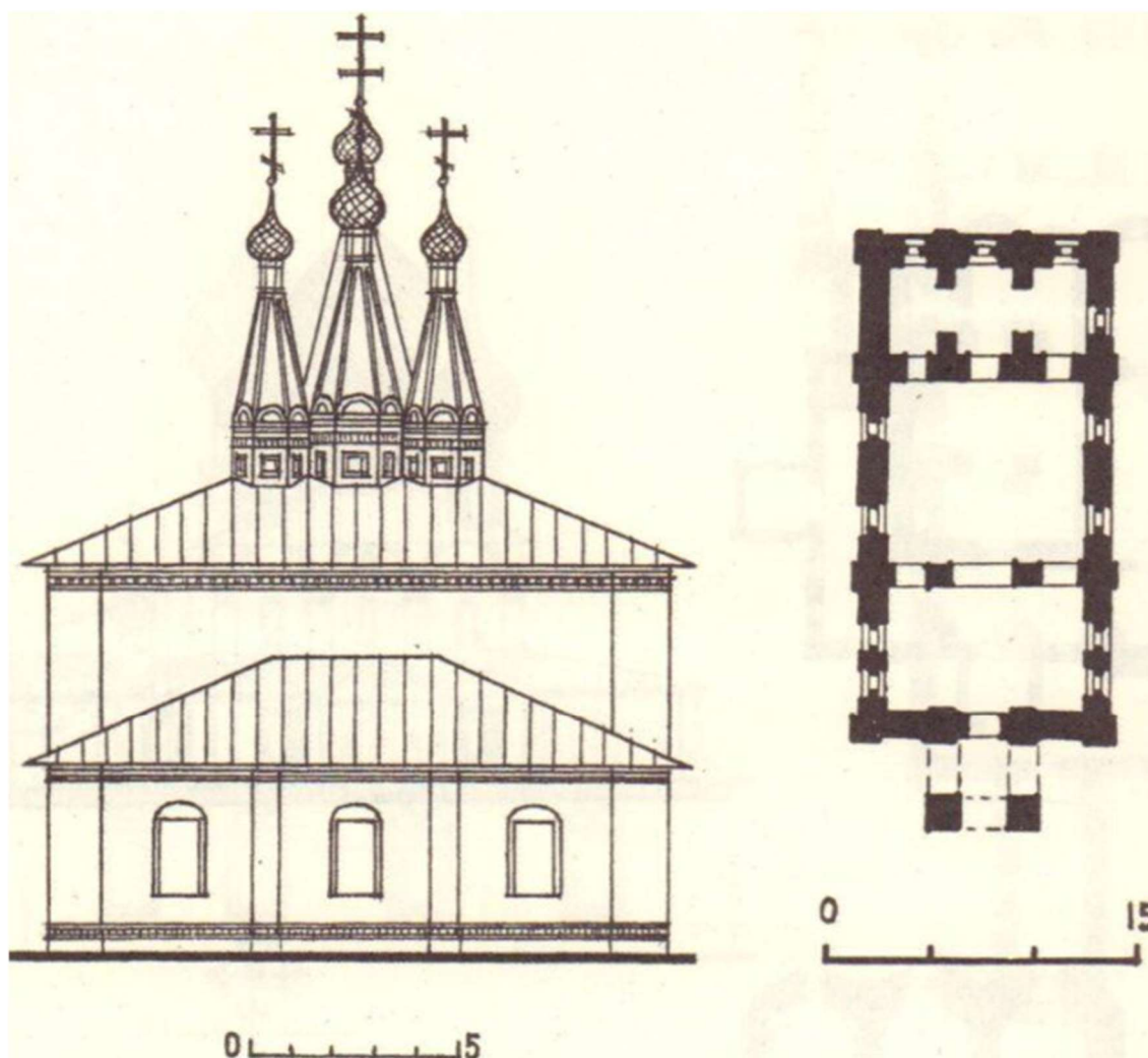
Церковь Владимирской иконы Божией Матери на Божедомке (1678 год): а - восточный фасад, б - план
