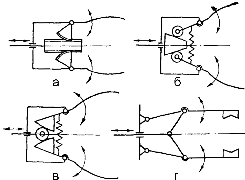
Кинематические схемы захватных устройств с плоскопараллельным движением губок: а – винтовое; б – с поступательным движением одной губки; в – с параллелограммным устройством
