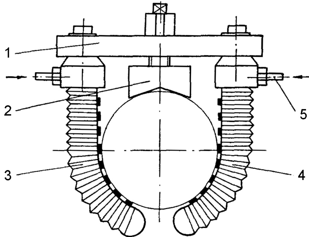
Захватное устройство с изгибающимися эластичными камерами 1 – корпус; 2 – базирующая призма; 3, 4 – эластичные камеры; 5 – трубопровод с пневмосистемой
