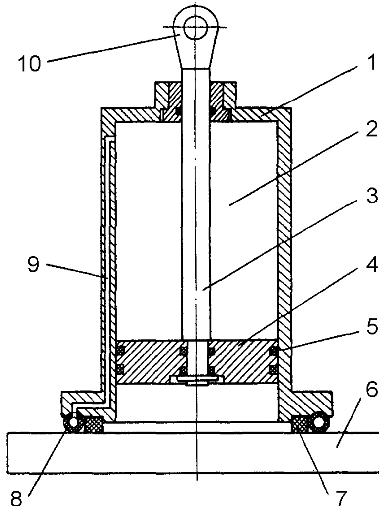
Безнасосное вакуумное устройство с поршнем 1 – цилиндрический корпус; 2 – центральная полость; 3 – боковая полость; 4 – поршень; 5 – уплотнения; 6 – объект манипулирования; 7 – эластичное уплотнение; 8 – основание; 9 – канал; 10 – серьга
