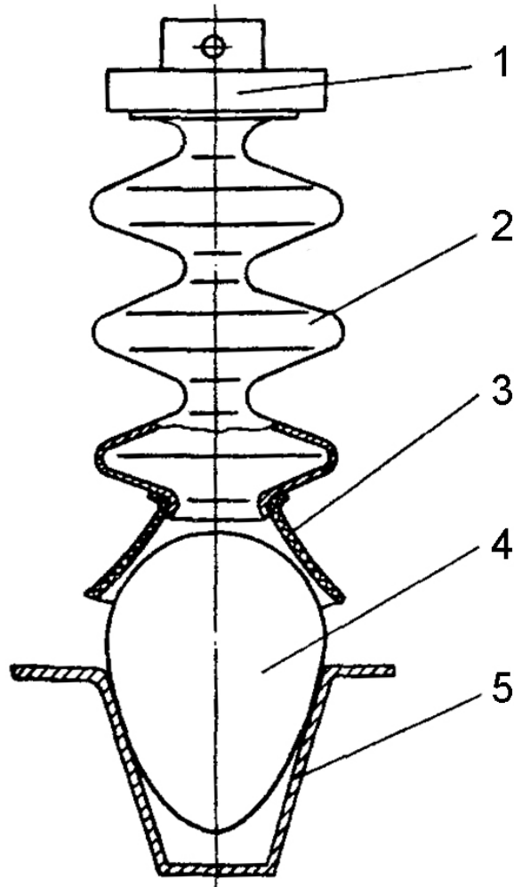
Безнасосное вакуумное захватное устройство 1 – корпус; 2 – гофрированная упругая труба; 3 – захватная эластичная горловина; 4 – объект манипулирования; 5 – ячейка
