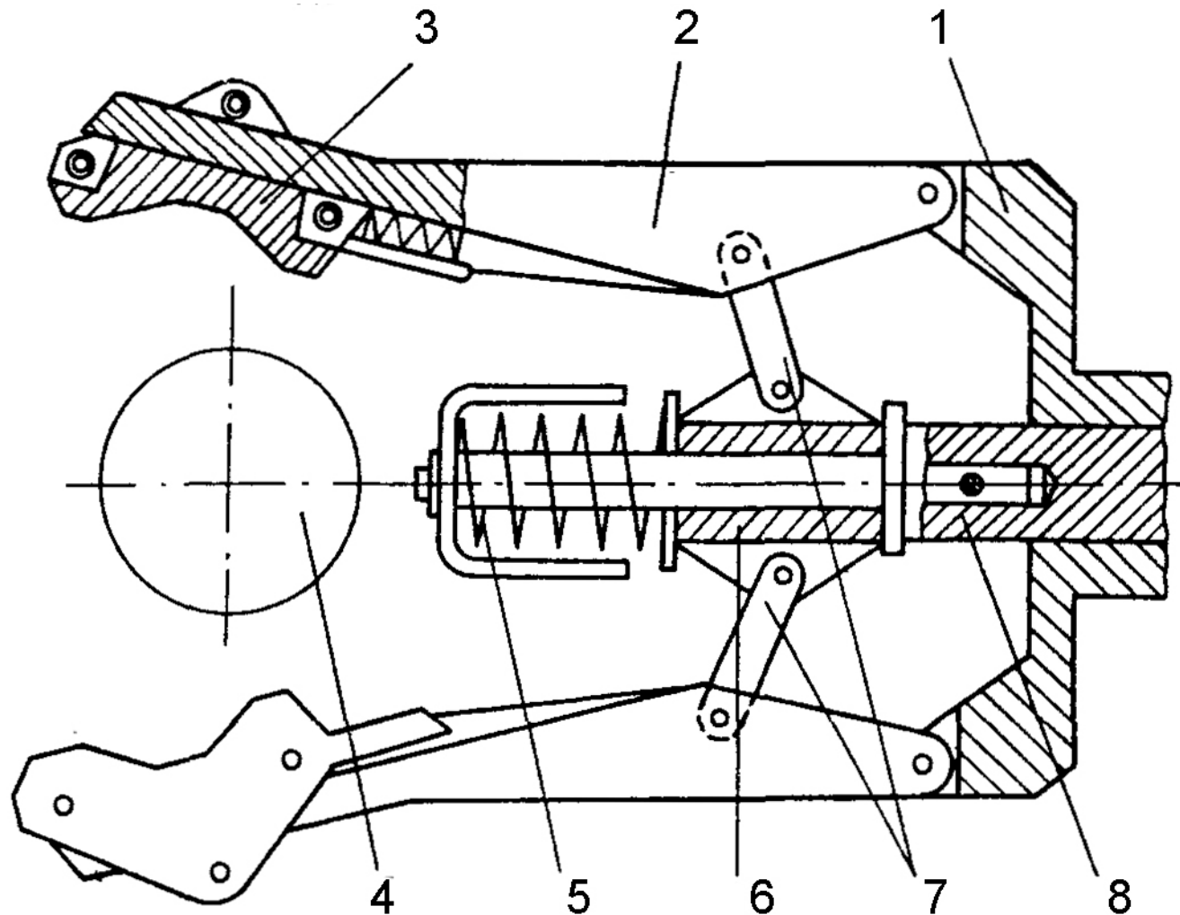
Механическое приводное захватное устройство с вращательным движением губок 1 – корпус; 2 – губки; 3 – захватные призмы; 4 – деталь; 5 – смягчающая пружина; 6 – ползун; 7 – рычаги; 8 – шток привода
