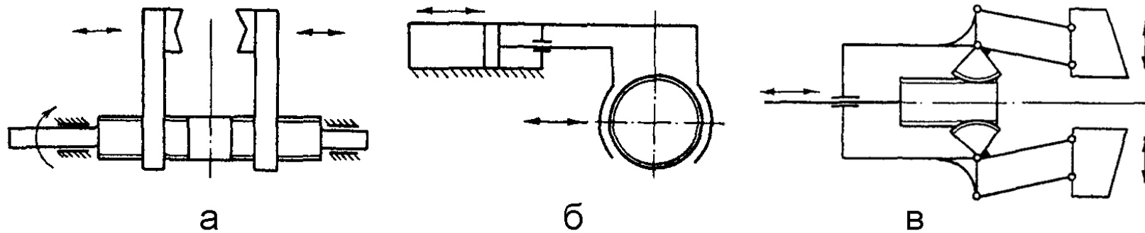
Кинематические схемы захватных устройств с плоскопараллельным движением губок: а – винтовое; б – с поступательным движением одной губки; в – с параллелограммным устройством
