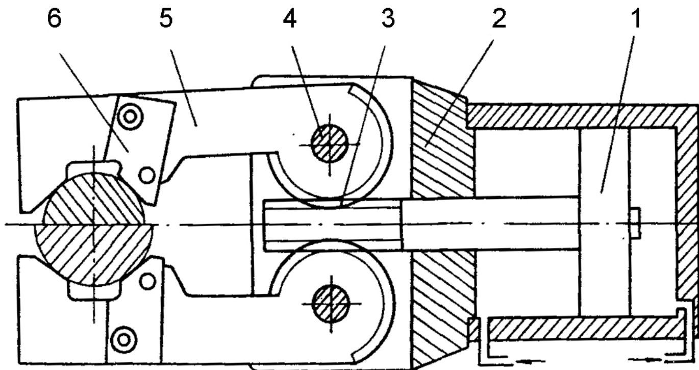
Механическое приводное захватное устройство с вращательным движением губок 1 – привод поступательного движения; 2 – корпус схвата; 3 – реечная передача; 4 – шарниры; 5 – корпус губок; 6 – подпружиненные сменные призмы
