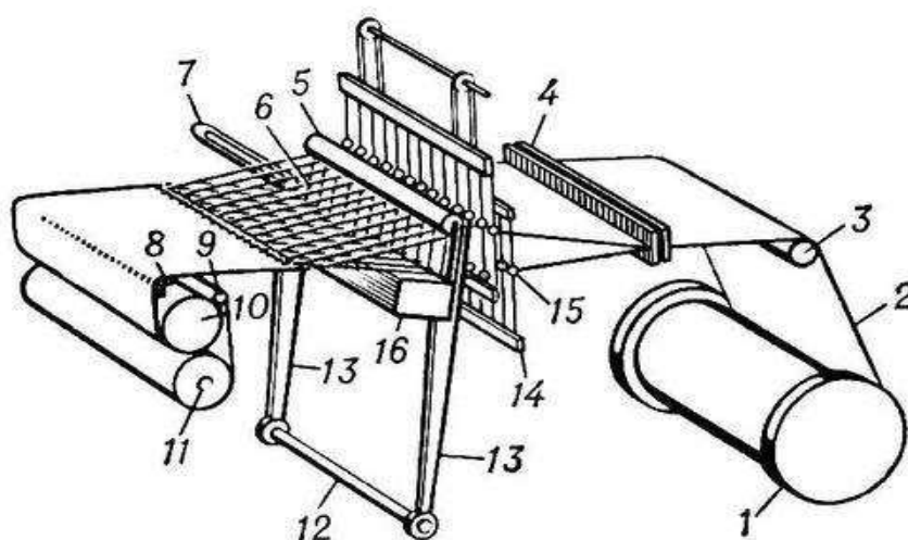
Рис. 13. Схема челночного ткацкого станка: 1 — навой; 2 — нити основы; 3 — скало; 4 — ламели; 5 — вершник; 6 — бердо; 7 — челнок; 8 — грудница; 9 — направляющий валик; 10 — вальян; 11 — товарный валик; 12 — подбатанный вал; 13 — лопасть батана; 14 — ремизка; 15 — глазок галева; 16 — батан
