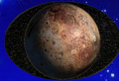
плутон
