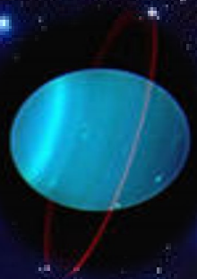
уран
