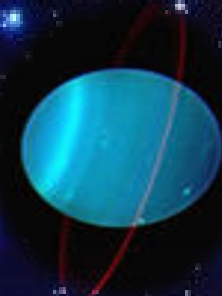
Уран
