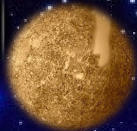
Меркурий
