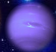
Нептун
