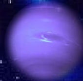
нептун
