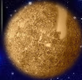
меркурий
