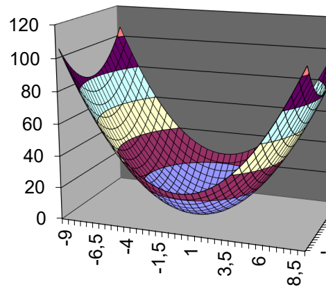
Параболоид вращения
